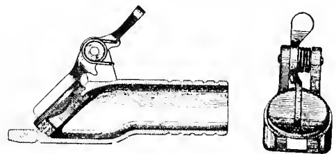
Fig. 1681. Longitudinal Section.
